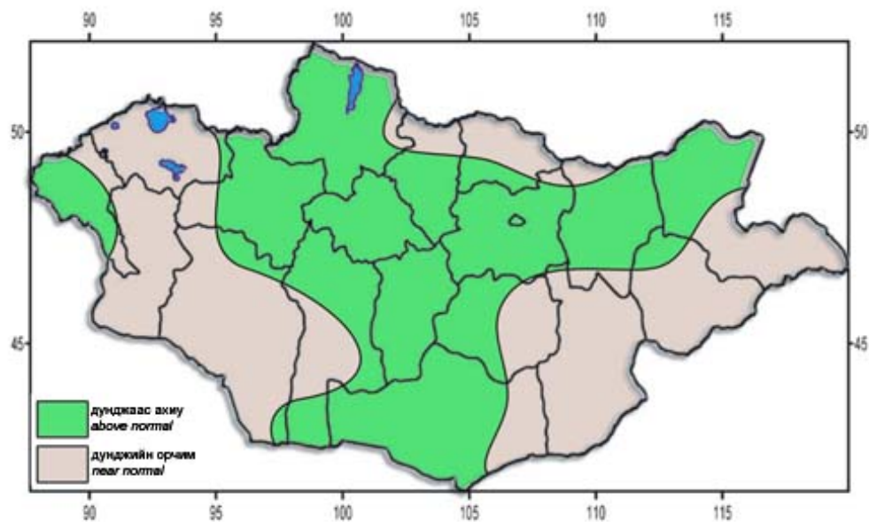
10 дугаар зураг. 2 дугаар сард орох хур тунадасны урьдчилсан мэдээ Precipitation forecast, February
