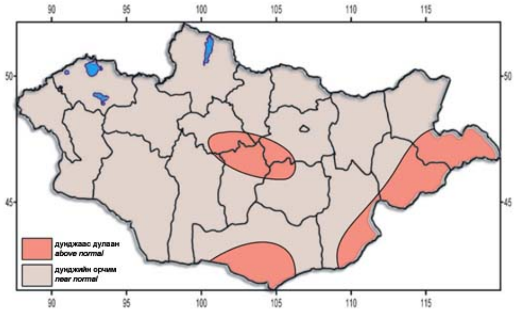
9 дүгээр зураг. 2 дугаар сарын агаарын температурын урьдчилсан мэдээ Air temperature forecast, February
